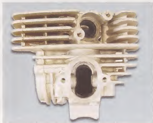
Culata de motor de cuatro tiempos
